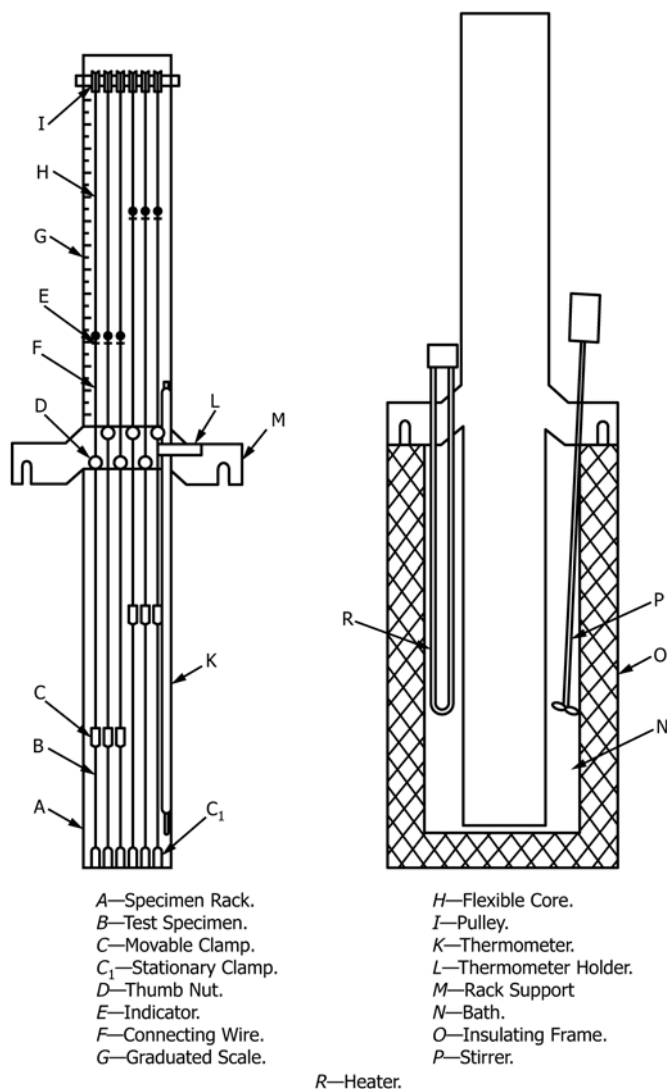
FIG. 1 Retraction Apparatus
