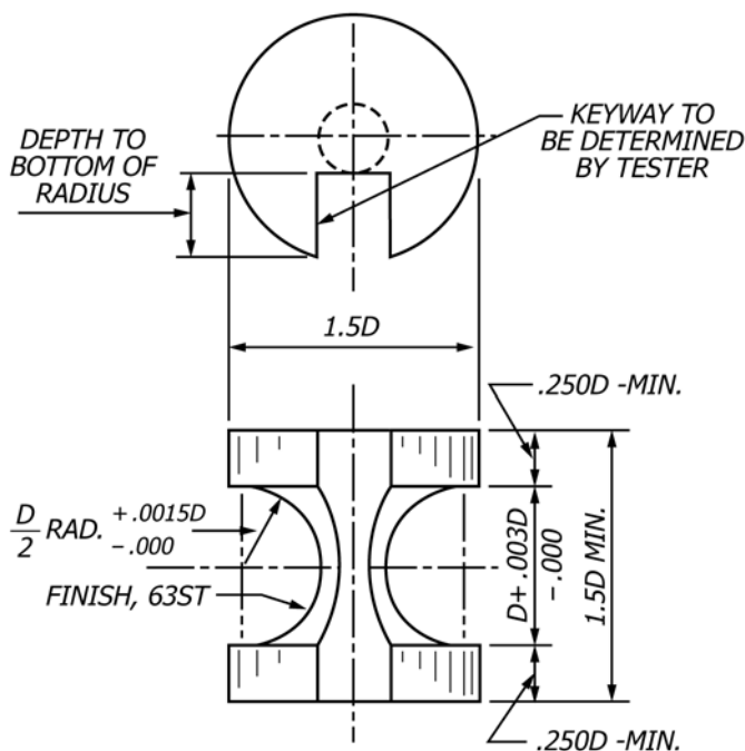
FIG. 2 Arbor Dimensions
