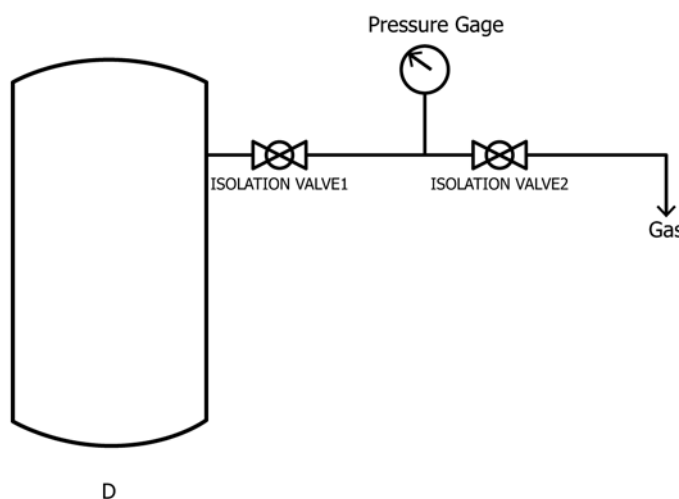
FIG. 1 Test Apparatus
